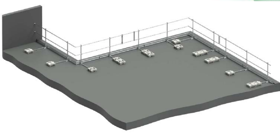
Ilustración 1: Sistema de protección lateral, tipo: BARRIER VARIO
